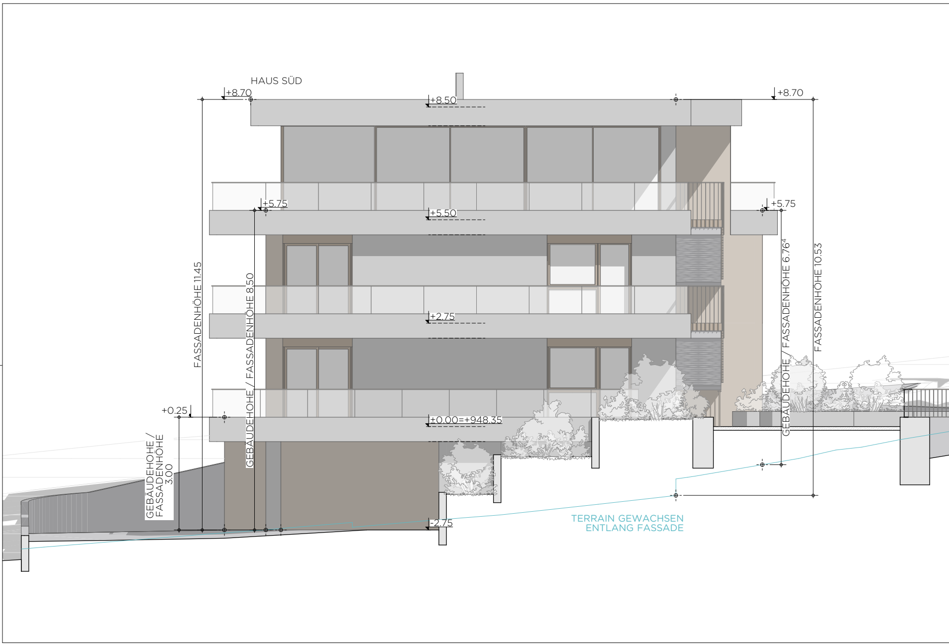
ANSICHT SÜD
