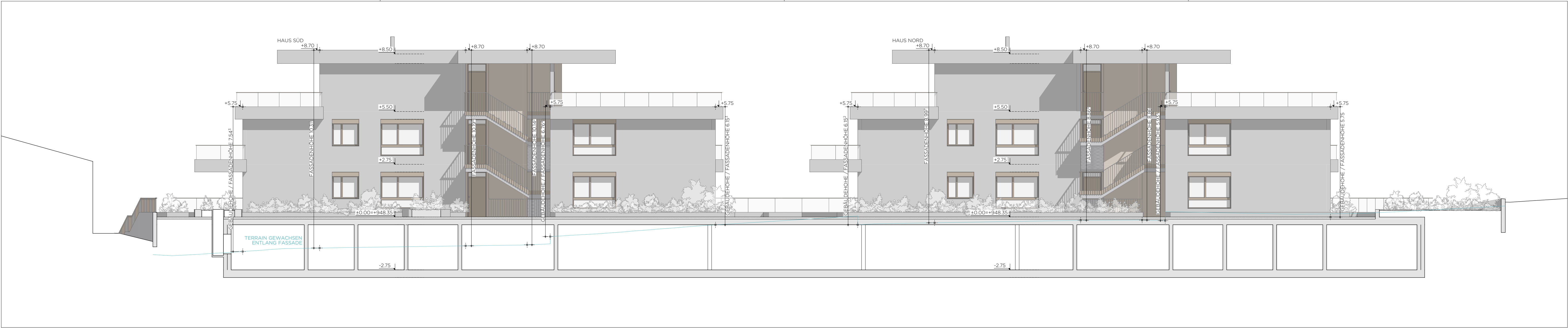
ANSICHT OST
