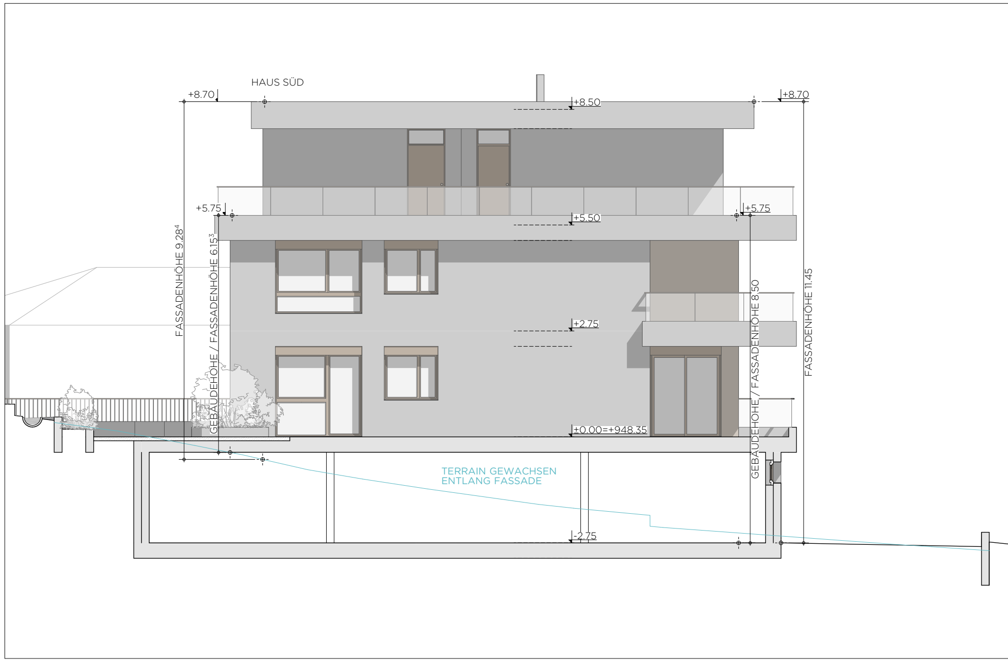
ANSICHT NORD
