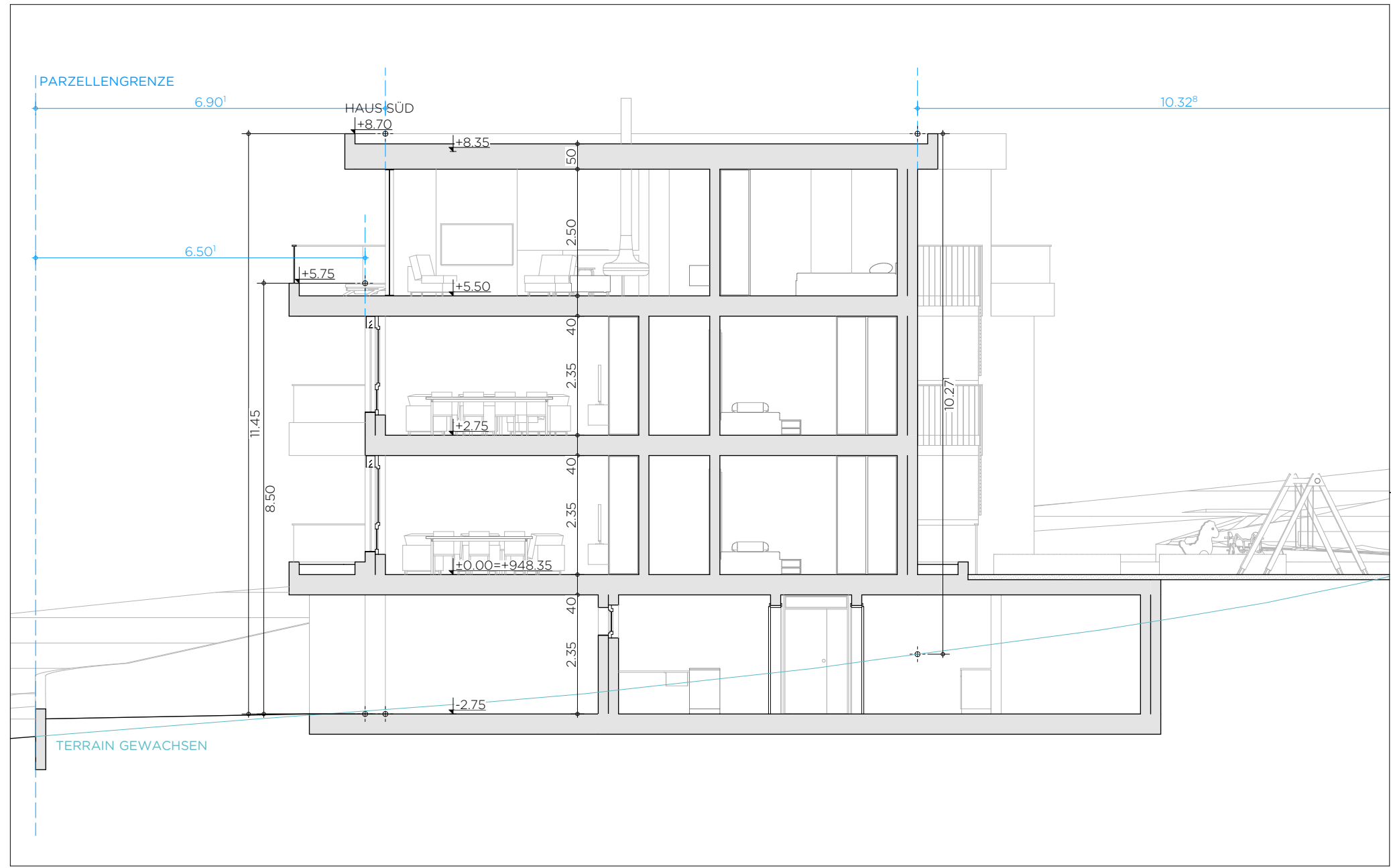
QUERSCHNITT 01
