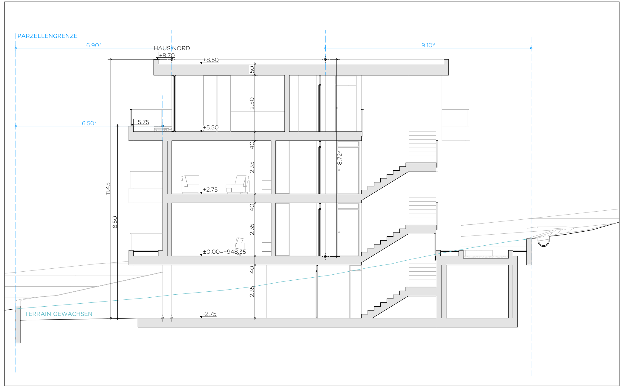
QUERSCHNITT 02
